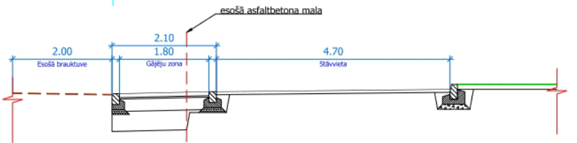
Griezums 1-1
